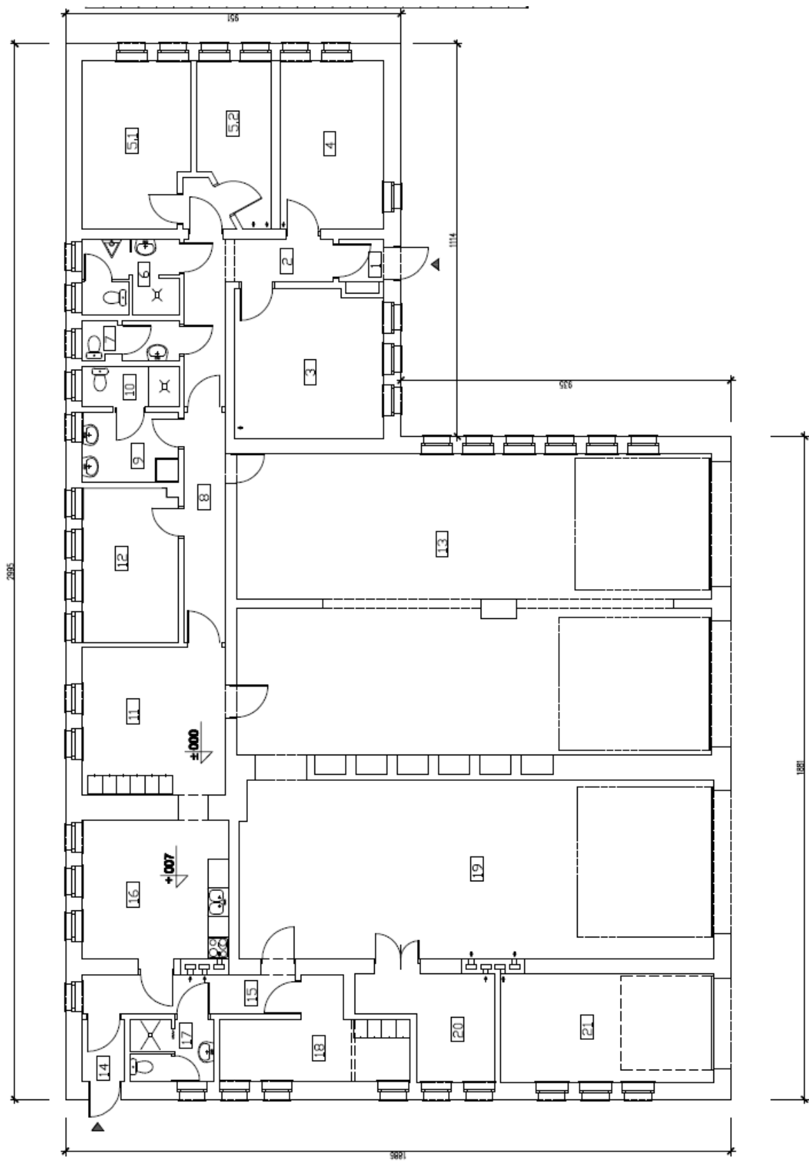
Rzut parteru
